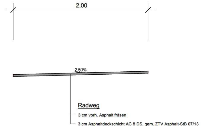
Regelquerschnitt 2 Radweg K 36 innerorts
