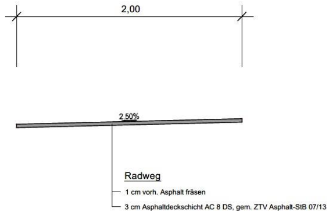
Regelquerschnitt 1 Radweg K 36 außerorts
