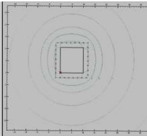
Abb. 2: Grafische Darstellung zur berechneten Reichweite des Absenktrichters bei einer definierten Fördermenge zur Grundwasserabsenkung
